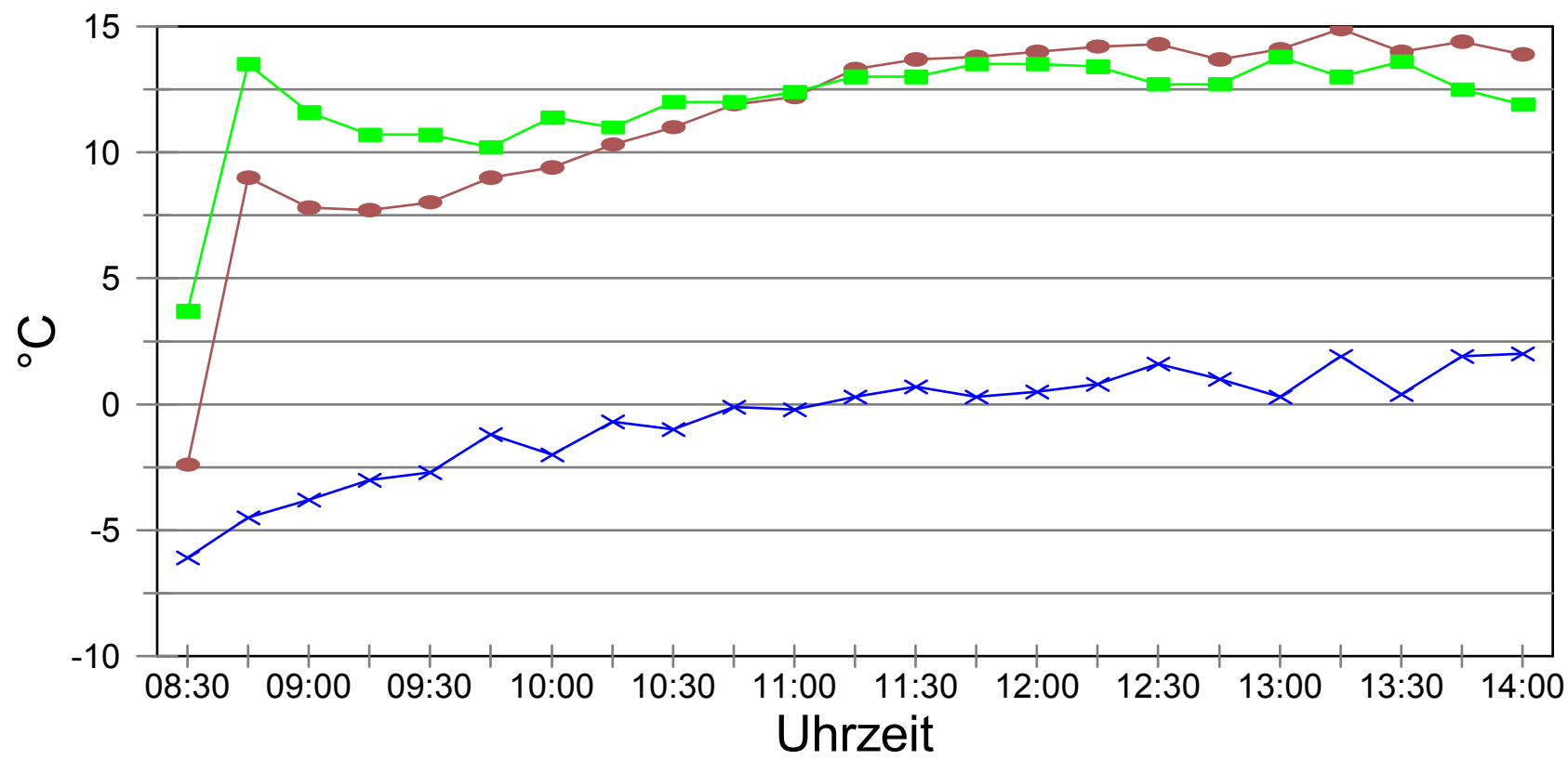
Temperaturmessung SV3, 28.02.05 Bochum - Süden - max Volumenstrom
